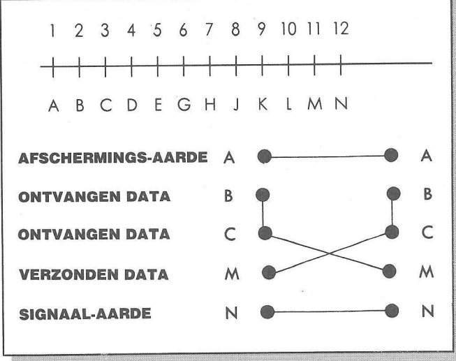
Afb. 1. Pennen van de gebruikerspoort
