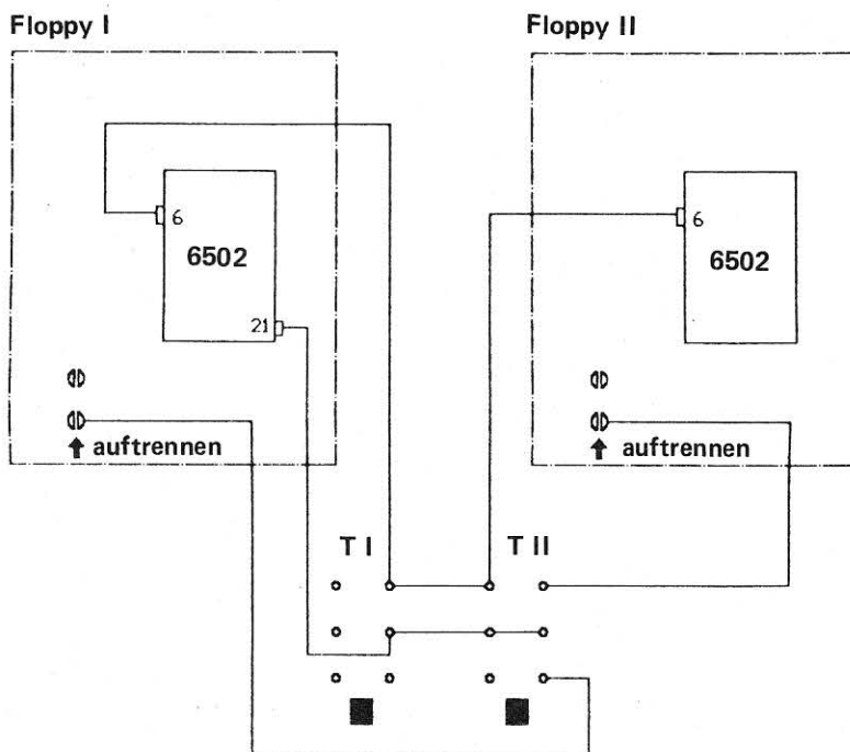
Abbildung 2: Der Aufbauplan
