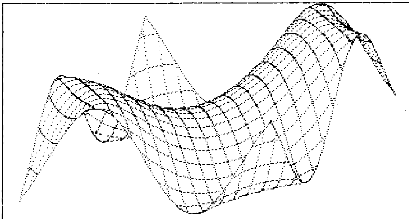
Figura 10.2 Grafico della funzione Z3 = \text{SIN}(X3 * Y3)
