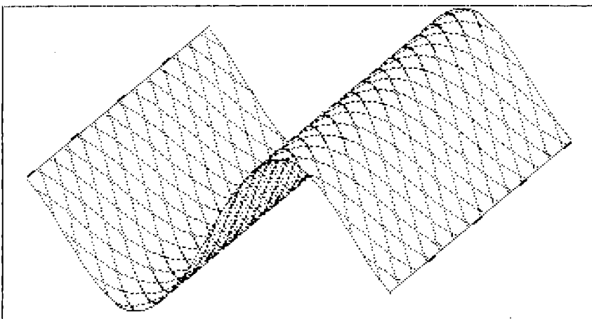
Figura 10.3 Grafico della funzione Z_3 = \text{SIN}(Y_3^2)
