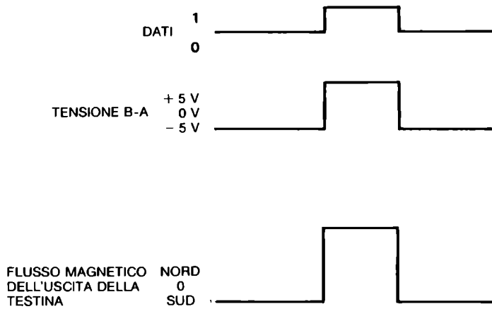
Figura 7.8b Livelli di tensione e magnetizzazione della testina del registratore
