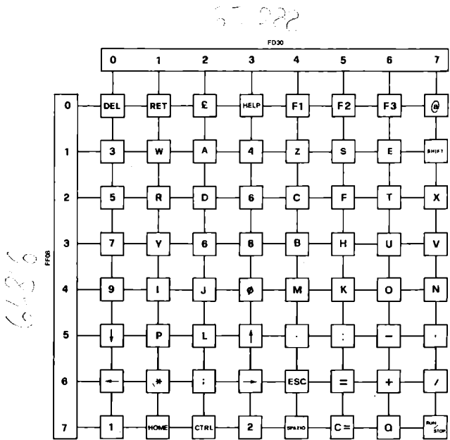
Figura 7.6 Organizzazione della tastiera
