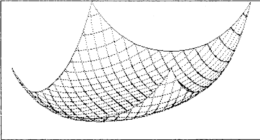
Figura 10.5 Grafico della funzione Z_3 = (X_3^3 + Y_3^3) * (X_3^3 + Y_3^3) / 32 - 1
