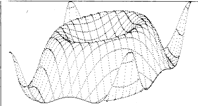
Figura 10.4 Grafico della funzione Z_3 = \text{SIN}(X_3^2 + Y_3^2)
