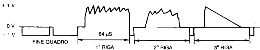
Figura 7.10 Segnale video per pilotare un monitor
