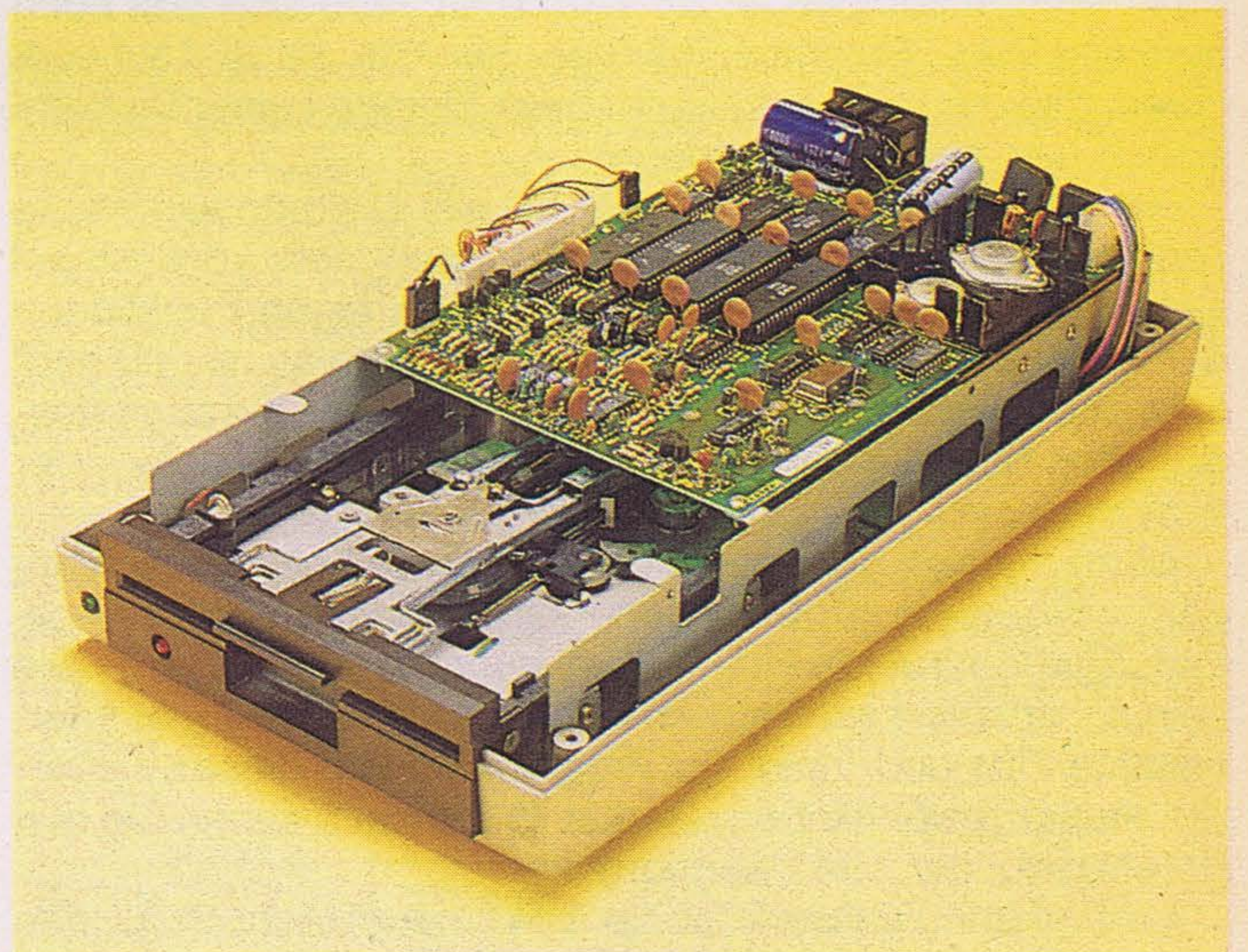
Bild 2. So sieht die 1541 von innen aus
