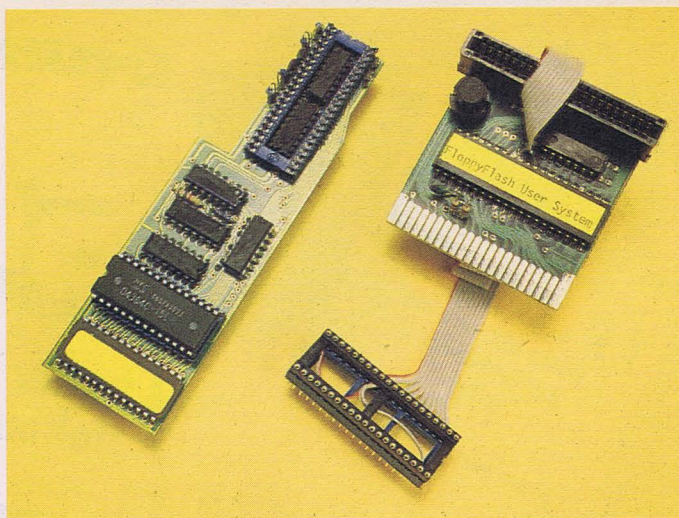
Bild 3. Professional Dos R4.0, das Aufbausystem. Hier bekommen alte Speeder neuen Glanz.
