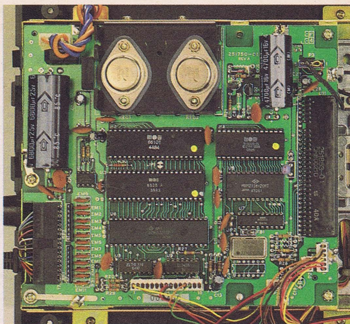
Bild 1. Die Platine der Floppy 1551. In der Mitte sehen Sie die Lötbrücke (JP1).
