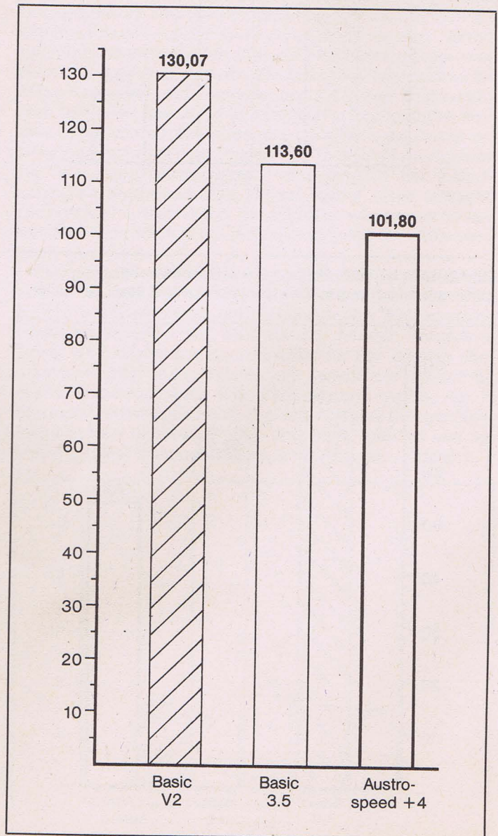
Bild 6. Da die Rechenroutinen des Interpreters benutzt werden, ist hier nicht viel gewonnen
