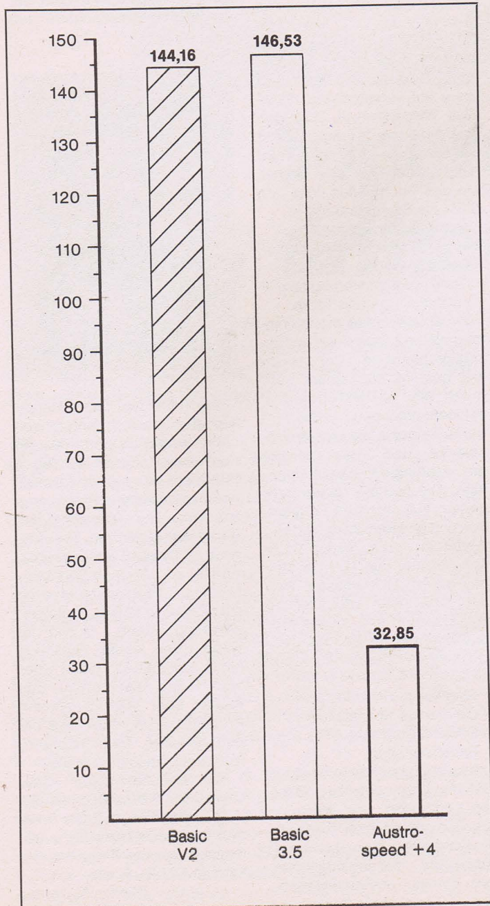
Bild 8. Die Durchschnittszeit für das Sortieren von 100 Zufallselementen mit Bubble-Sort
