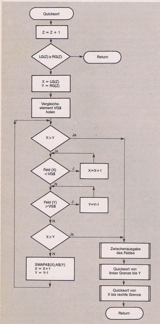
Bild 10. Die Arbeitsweise von Quicksort
